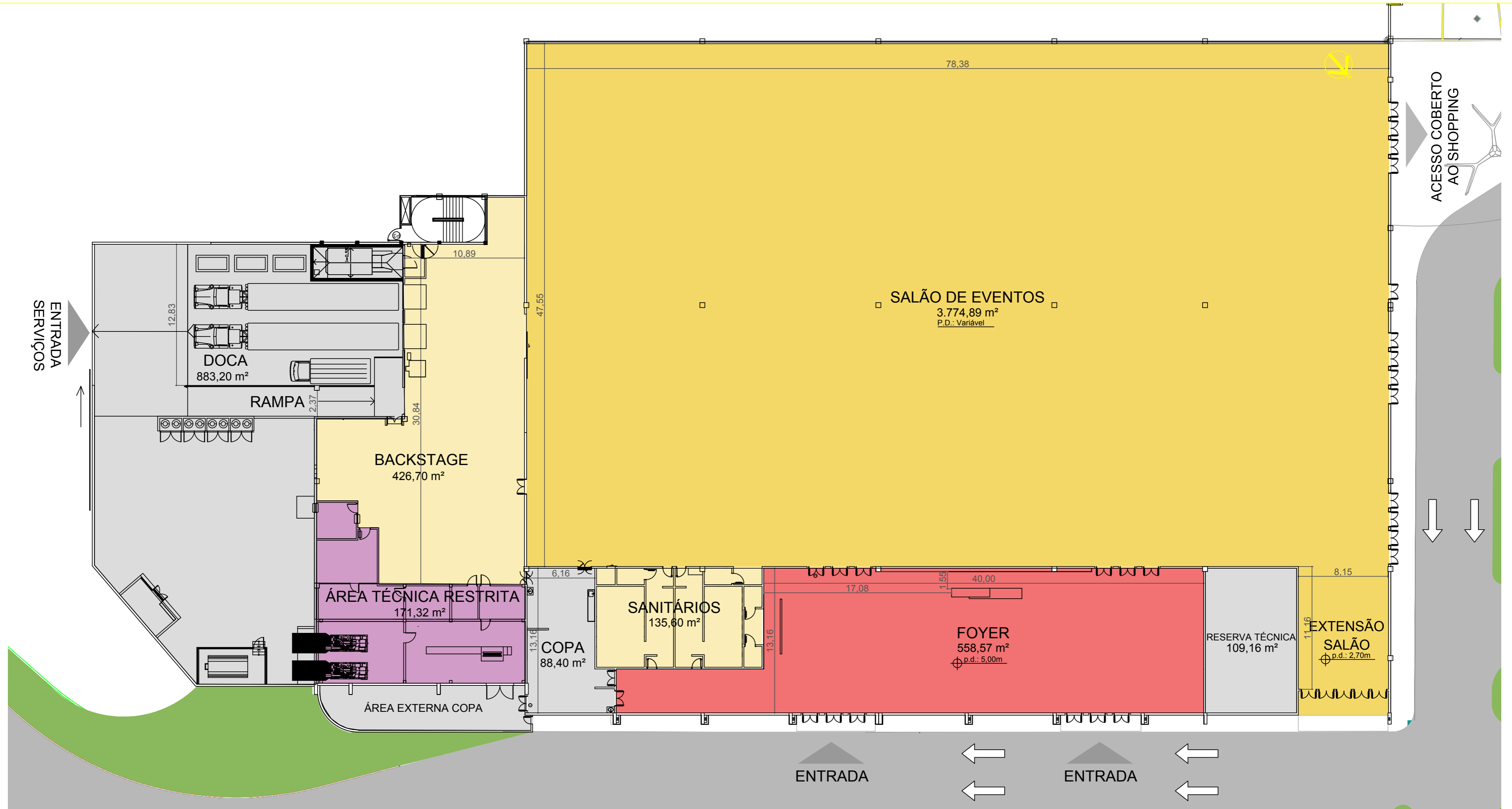
PLANTA BAIXA - CENTRO DE EVENTOS
